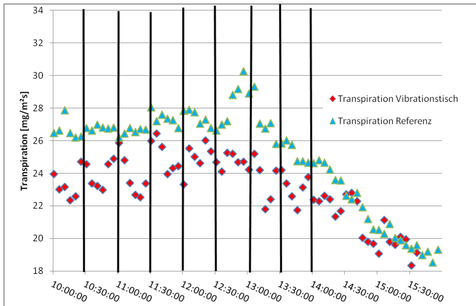
Abb. 35: Verlauf der Transpiration von Euphorbia pulcherrima 'Bella Italia Red' der Vibrationsvariante 15 Hz (2x10 min/h, zwischen 6-18 Uhr) und der Kontrolle (unbehandelt, ohne Wuchshemmstoffe), senkrechte Linien zeigen den Beginn der Vibrationsbehandlung, 11.12.2013
