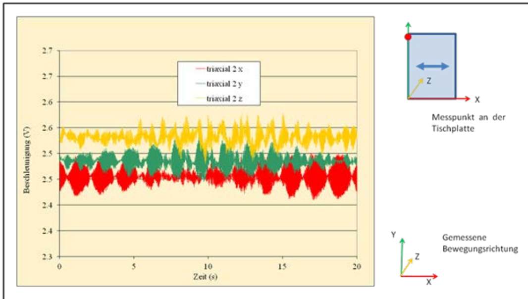
Abb. 3: Beschleunigung in x-, y- und z- Richtung am Rahmen des Vibrationstisches, Frequenz - 50 Hz (Vibrationstisch mit Gummi-Metall-Puffern)
