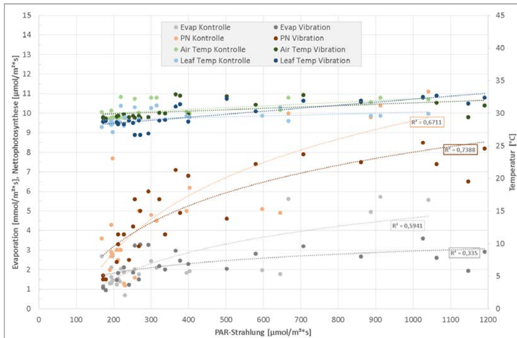
Abb. 36: Gaswechsellmessungen (CIRAS) an Ocimum basilicum 'Siam Queen' (Thaibasilikum) im Wechsel an je 7 vibrierten Pflanzen und 7 Kontrollpflanzen, (Evap – Transpiration, PN – Nettophotosynthese, Air Temp – Lufttemperatur, Leaf Temp – Blatttemperatur), 08.07.2016
