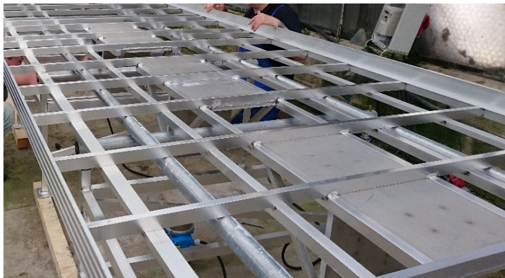
Abb. 8: Drei Aluminium-Montageplatten zur Motorenbefestigung, 2016 Abb. 9: Unwuchtmotoren zur Vibrationserzeugung
