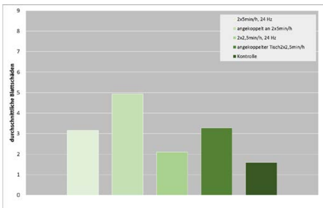
Abb. 30: Einfluss von unterschiedlichen Vibrationsdauern und gekoppelten Tischen (mit und ohne Antrieb) im Vergleich zur Kontrolle auf die durchschnittlichen Blattschäden von Ocimum basilicum 'Edwina' (1-keine Schäden, 3-sehr leichte Blattschäden, 5-mittlere Schäden, 7-starke Blattschäden, 9-sehr starke Blattschäden), 2015
