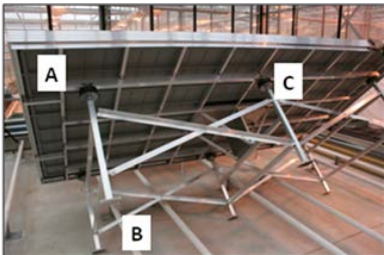
Abb. 1. Vibrationstisch mit Gummi-Metall-Puffern (verbiegungssteife Tischplatte (A), verstärkte und schwingungsgedämmte Unterkonstruktion (B), massive Montage-platte (C))
