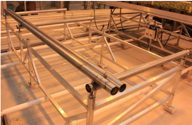
Abb. 6: Unterkonstruktion Vibrations-Rolltisch
