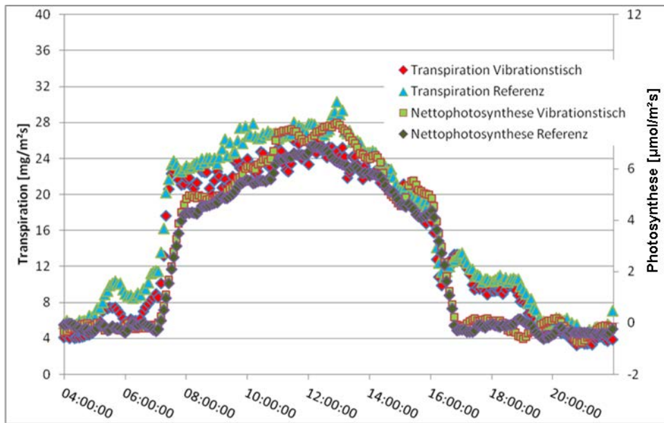
Abb. 33: Tagesverlauf der Nettophotosynthese und der Transpiration von Euphorbia pulcherrima 'Bella Italia Red' der Vibrationsvariante 15 Hz (2x10 min/h, zwischen 6-18 Uhr) und der Kontrollvariante (unbehandelt, ohne Wuchshemstoffe), 11.12.2013
