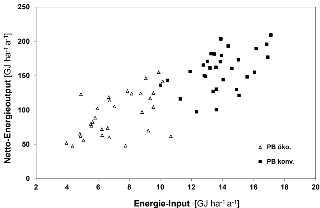
Abbildung 5.3-1: Beziehung zwischen dem Energie-Input und dem Netto-Energieoutput im Pflanzenbau.
