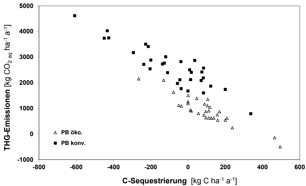
Abbildung 5.3-4: Beziehung zwischen der C-Sequestrierung und den flächenbezogenen Treibhausgasemissionen im Pflanzenbau.
