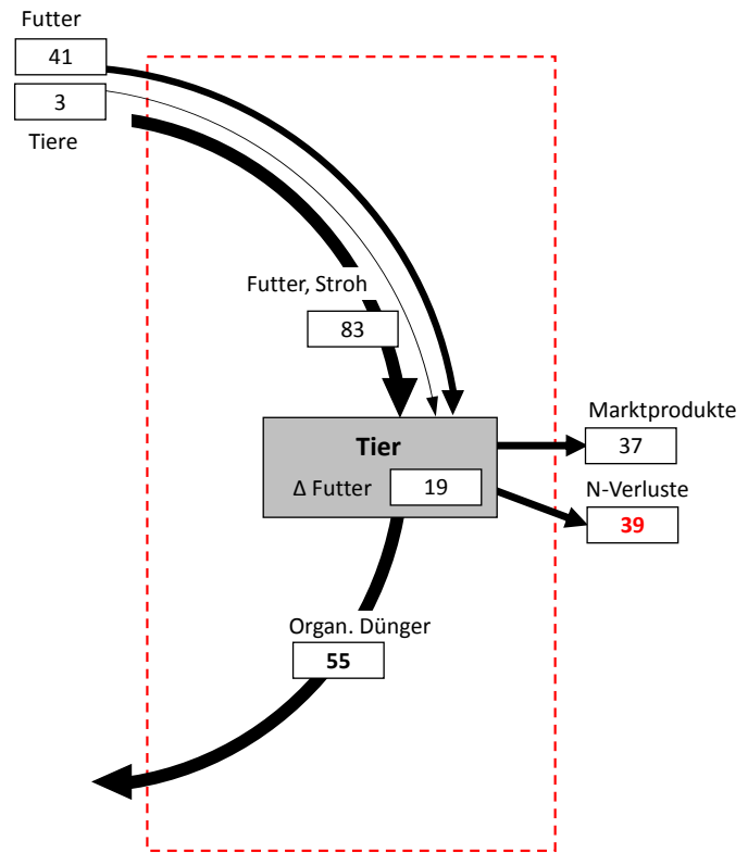
Abbildung 5.4-3: Stallbilanz ( \text{kg N ha}^{-1} \text{a}^{-1} ), Pilotbetrieb PB 68 [N-Saldo = 39 \text{ kg N ha}^{-1} \text{a}^{-1} , N-Effizienz I = 35 % (ohne org. Dünger)] [N-Effizienz II = 85 % (mit org. Dünger)].
