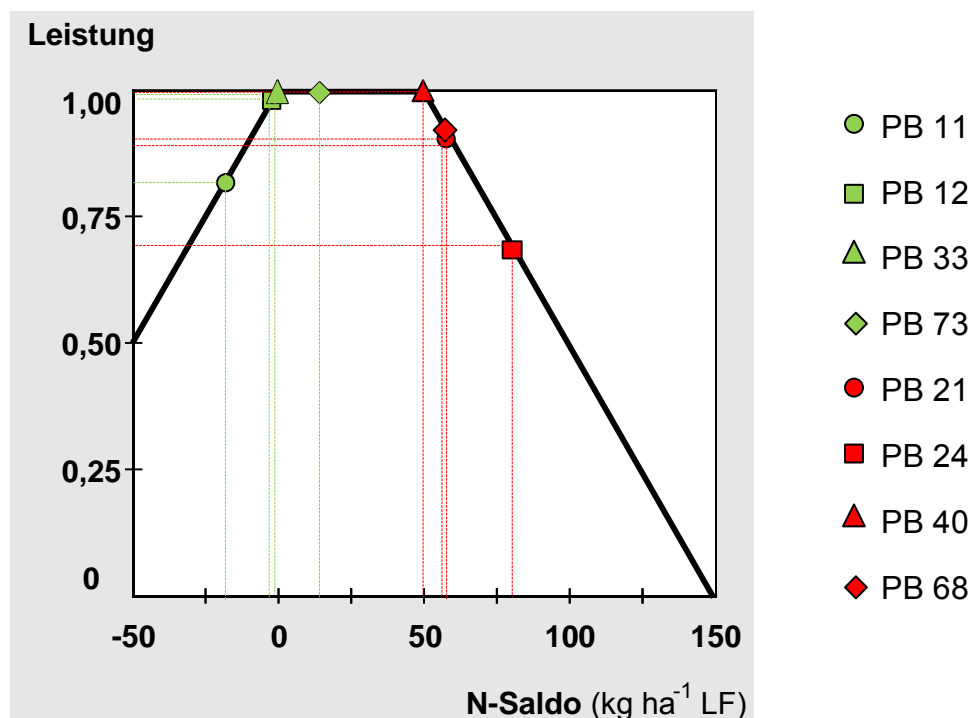
Abbildung 5.4-5: Bewertungsfunktion Stickstoffsaldo 2 , Bewertung der flächenbezogenen N-Salden der Pilotbetriebe.
