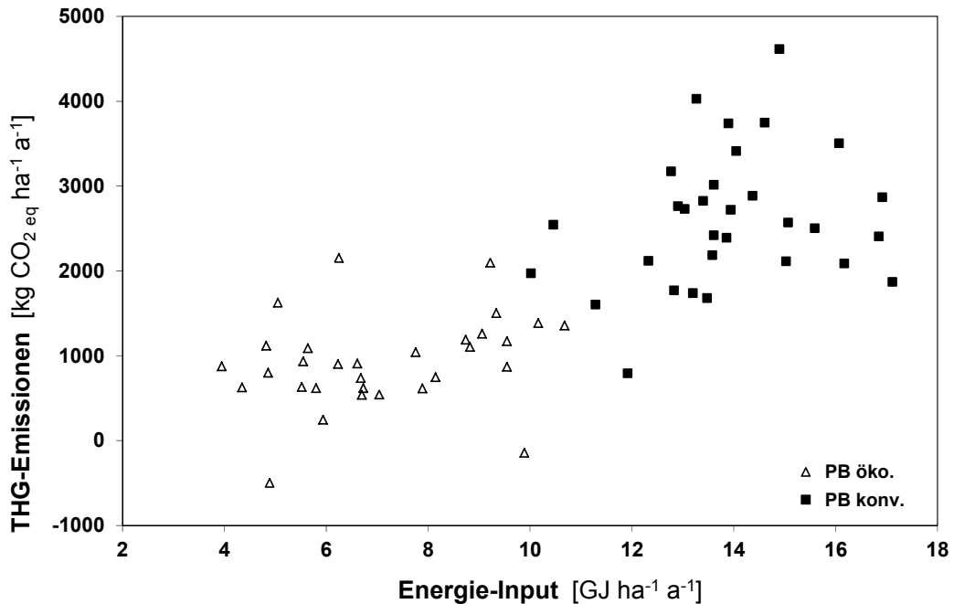
Abbildung 5.3-3: Beziehung zwischen dem Energie-Input und den flächenbezogenen Treibhausgasemissionen im Pflanzenbau.
