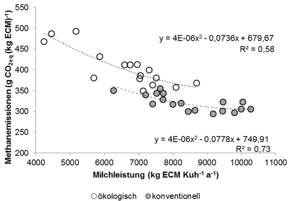
Abbildung 5.1-3: Methanemissionen der Milchproduktion in Abhängigkeit von der Milchleistung.
