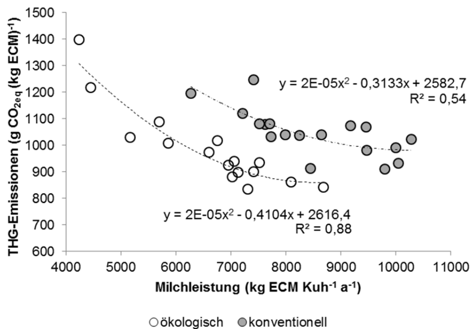
Abbildung 5.1-4: THG-Emissionen der Milchproduktion in Abhängigkeit von der Milchleistung.
