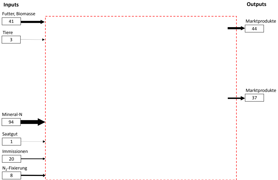
Abbildung 5.4-2: Hoftorbilanz ( \text{kg N ha}^{-1} \text{a}^{-1} ), Pilotbetrieb PB 68 (N-Saldo = 86 \text{ kg N ha}^{-1} \text{a}^{-1} , N-Effizienz = 49 %).
