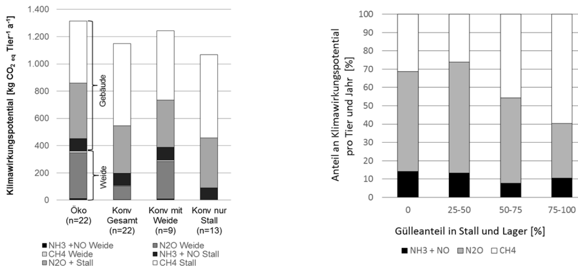
Abbildung 5.2-1: Klimawirkungspotential aus Exkrementen der Milchkühe pro Kuh auf den Pilotbetrieben (Mittelwerte der Jahre 2008 bis 2010).
