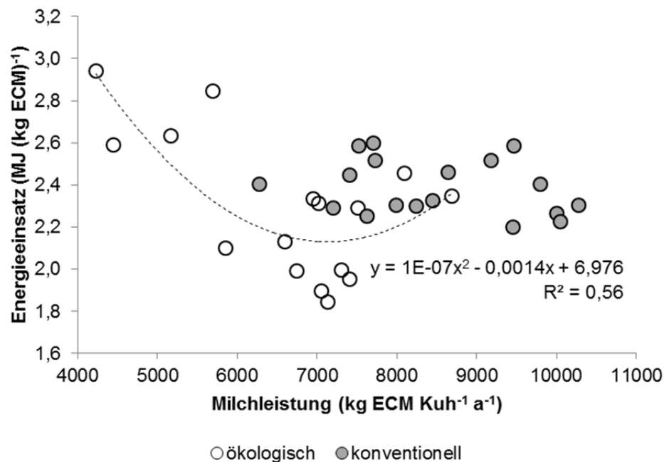
Abbildung 5.1-2: Energieeinsatz für die Milchproduktion in Abhängigkeit von der Milchleistung.
