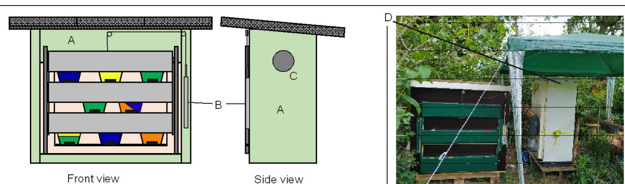
Abbildung 4: Styroporbox zur Kühlung kleiner Begattungseinheiten auf Imkerständen A: Styrodur-Korpus, B: Gegengewicht für Falltür; C: Loch für Kaltluftzufuhr; D: Gefrierschrank für Kälterzeugung
