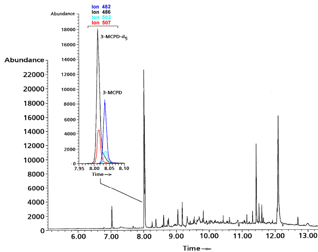
Abbildung 2.3: Ionenchromatogramm einer dotierten Rattenblutprobe (20 ng/ml 3-MCPD) nach Aufarbeitung und Derivatisierung (HFBA Derivat).
