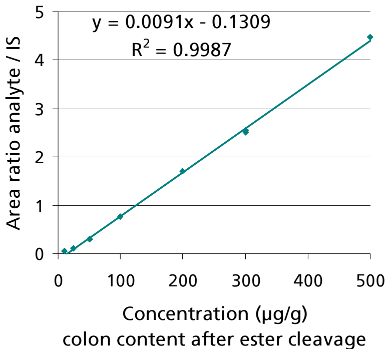
Abbildung 2.6: Kalibriergerade für 3-MCPD-ester im Rattendickdarminhalt nach Aufarbeitung (organische Phase), Esterspaltung und Derivatisierung (PBA-Derivat von 3-MCPD) (Konzentrationsbereich 10-500 µg/g 3-MCPD-ester, 100 µg/g interner Standard.)
