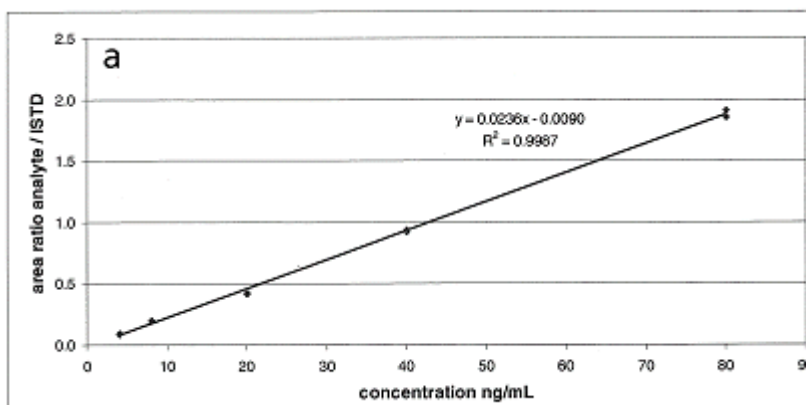
Abbildung 2.4: Kalibriergerade für 3-MCPD (HFBA-Derivat) in Rattenblut (Konzentrationsbereich 4-80 ng/ml 3-MCPD, 40 ng/ml 3-MCPD-d 5 )
