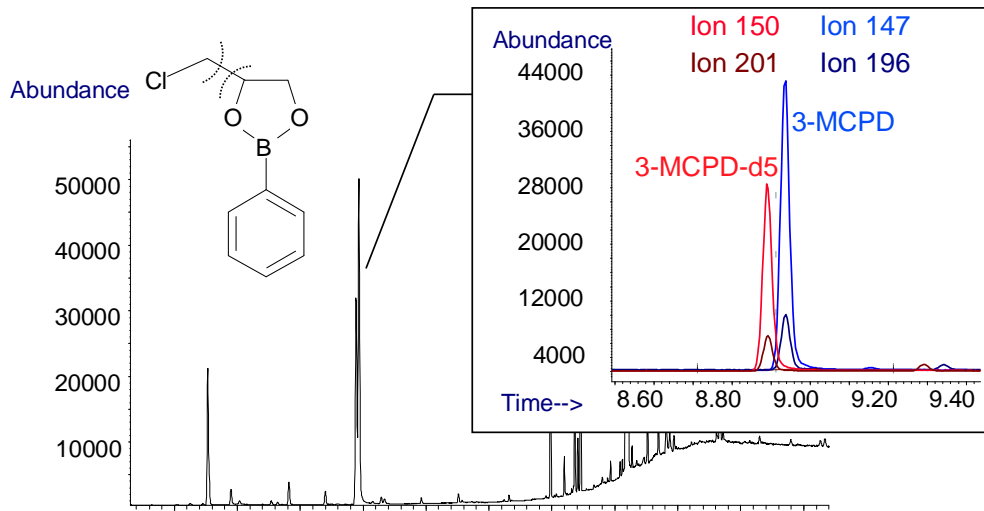
Abbildung 2.5: GC-MS (EI) Chromatogramm einer realen Probe der Rattendünndarmwand nach Aufarbeitung (organische Phase), Esterspaltung und Derivatisierung (PBA-Derivat von 3-MCPD).
