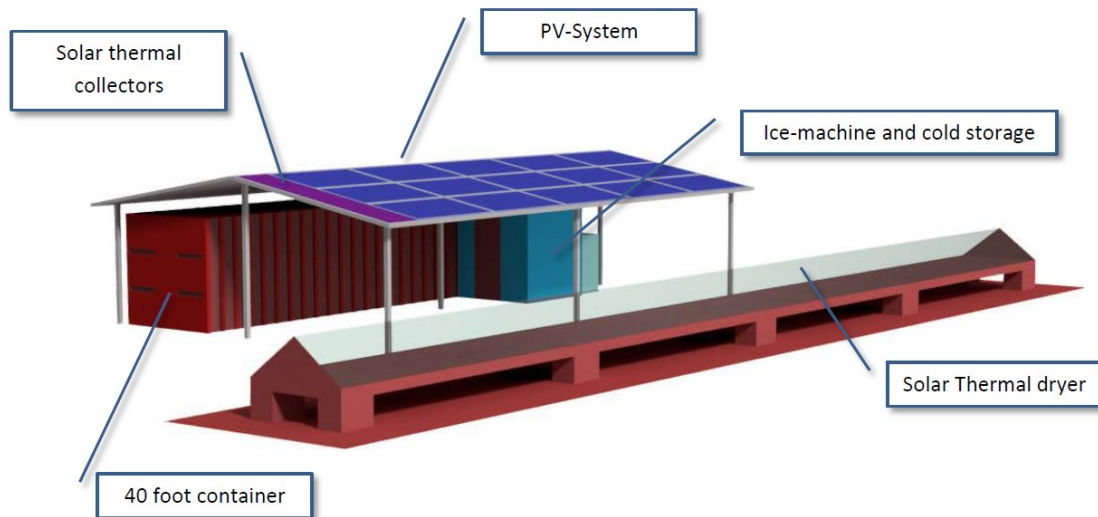
Abb. 3: Systemschema mit Fotovoltaik-Anlage, Solarkollektoren, 40-Fuß-Container, Eismaschine und kleinem Kühlraum für das Flake-Eis sowie solarthermischer Trockner
