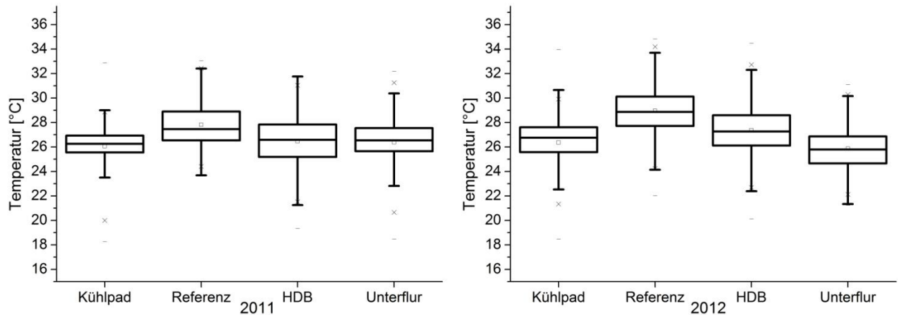
Abb. 46: Temperaturwerte im Abteil bei einer Außentemperatur >22^{\circ}\text{C} . Links: Jahr 2011 Jan. – Dez. ( n > 652 h), rechts: Jahr 2012 Jan. – Sep. ( n > 700 h). (HDB = Hochdruckbefeuchtung)
