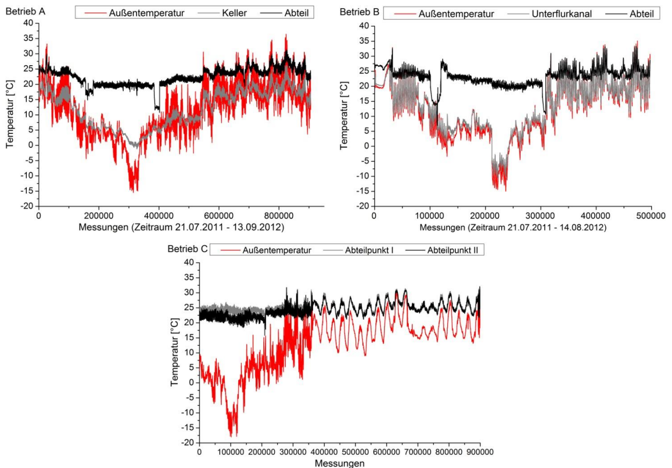
Abb. 61: Verlauf der Temperaturwerte über den Untersuchungszeitraum auf den jeweiligen Praxisbetrieben. Links oben: Betrieb A (Erdwärmetauscher), rechts oben: Betrieb B (Unterflurzuluft), unten: Betrieb C (Hochdruckbefeuchtung)
