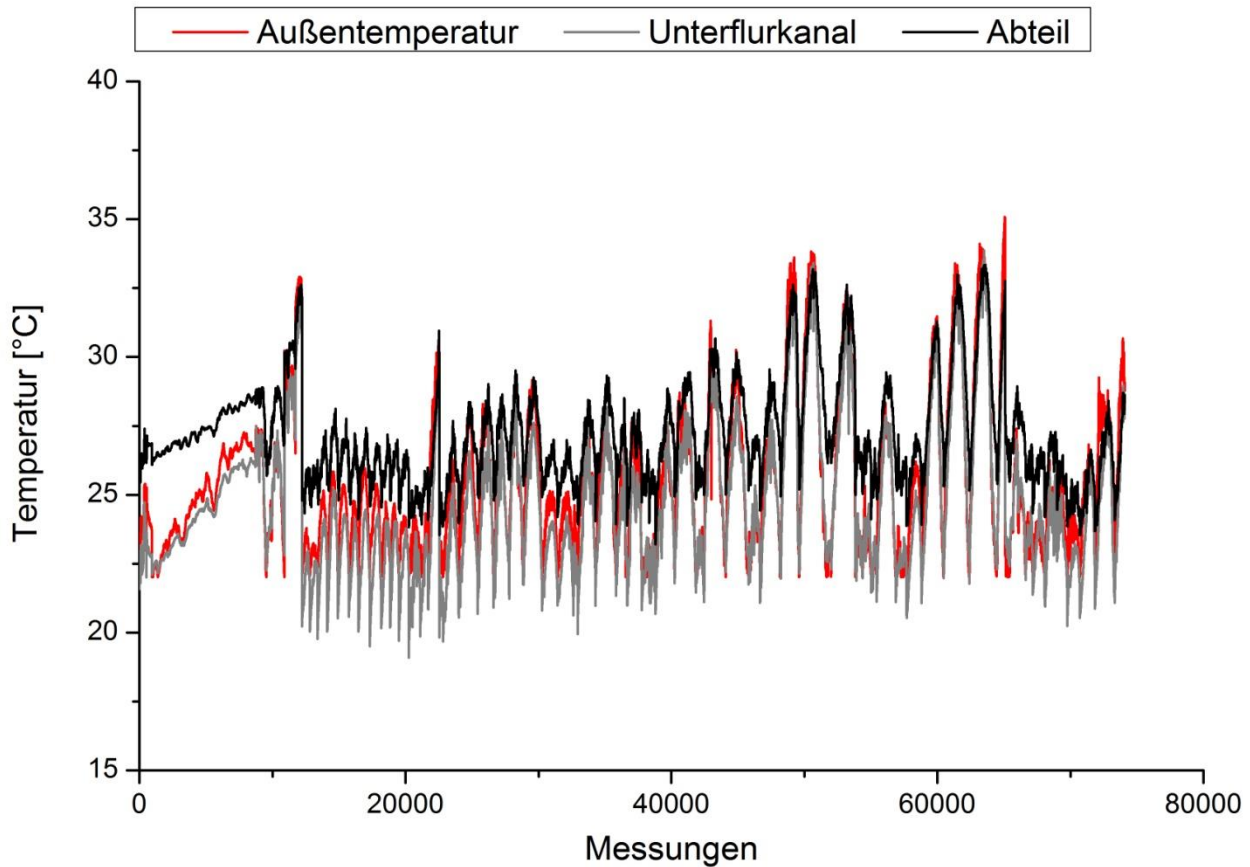
Abb. 64: Temperaturmesswerte bei einer Außentemperatur >22^{\circ}\text{C} bei dem Betrieb B (Unterflurzulufführung).
