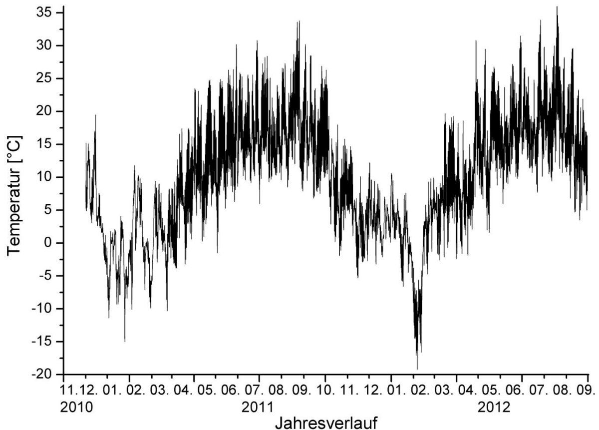
Abb. 39: Temperaturverlauf des Außenfühlers am Maststall der LSZ Boxberg.
