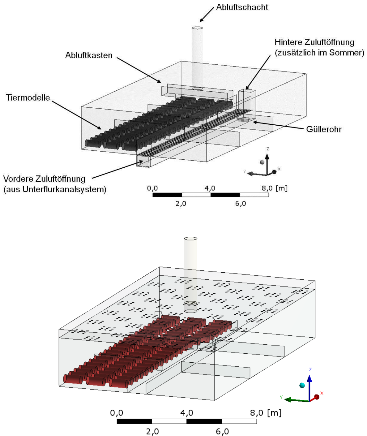
Abb. 37: Modell des Abteils mit Unterflurzuluft (oben) und des Abteils mit Porendecken- zuluft (unten) (ADRION, 2013)
