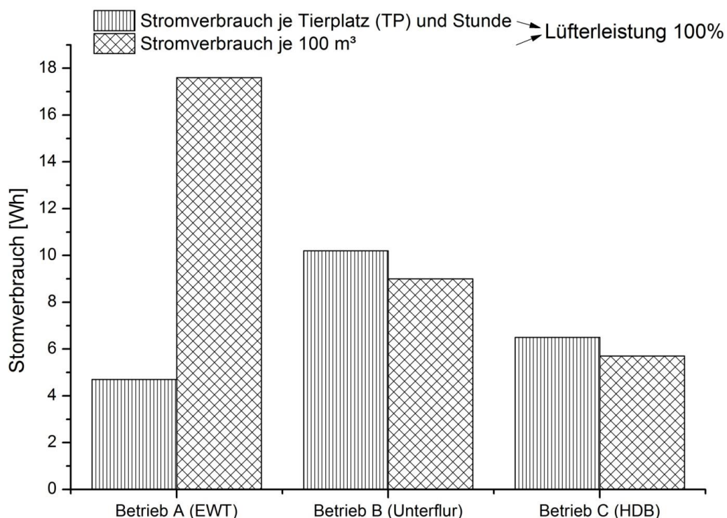
Abb. 83: Vergleich des Stromverbrauchs der Ventilatoren bei 100% Lüfterleistung für eine Stunde mit dem Bezug auf den Tierplatz und als weiterer Vergleich der Stromverbrauch bei 100% Lüfterleistung für die Förderung von 100 m 3 Luft von den Praxisbetrieben Erdwärmetauscher (EWT), Unterflurzuluft und Hochdruckbefeuchtung (HDB).
