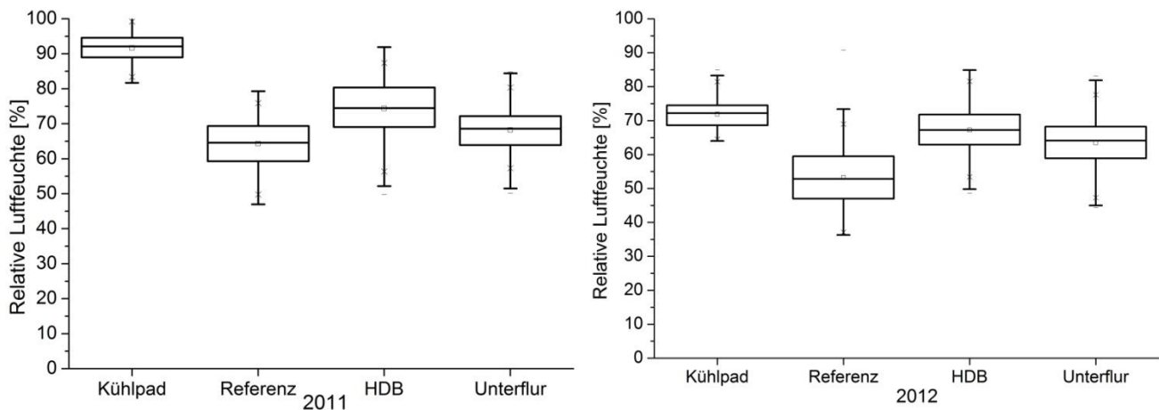
Abb. 51: Relative Luftfeuchtigkeitswerte über die zwei wärmsten Zeiträume. Links: 18.08. – 26.08.2011 n >25000; rechts: 17.08. – 21.08.2012 n >14000
