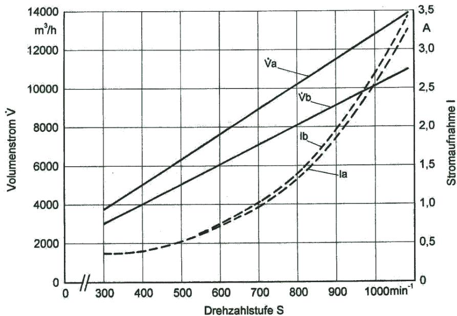
Abb. 14: Volumenstrom und Stromaufnahme bei: 300 bis 1100 \text{U min}^{-1} , (a) 50 Pa - und (b) 105 Pa Widerstand (NIEDHAMMER, 2000) (---- Volumenstrom - - - - Stromaufnahme)
