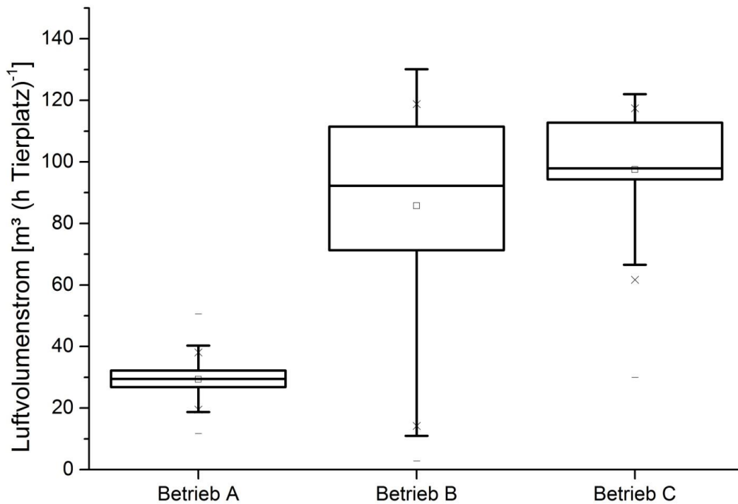
Abb. 66: Luftvolumenstromwerte je Tierplatz von den Betrieben A (Erdwärmetauscher), B (Unterflur) und C (Hochdruckbefeuchtung) bei einer Außentemperatur von >22^{\circ}\text{C} . ( n > 74000 )
