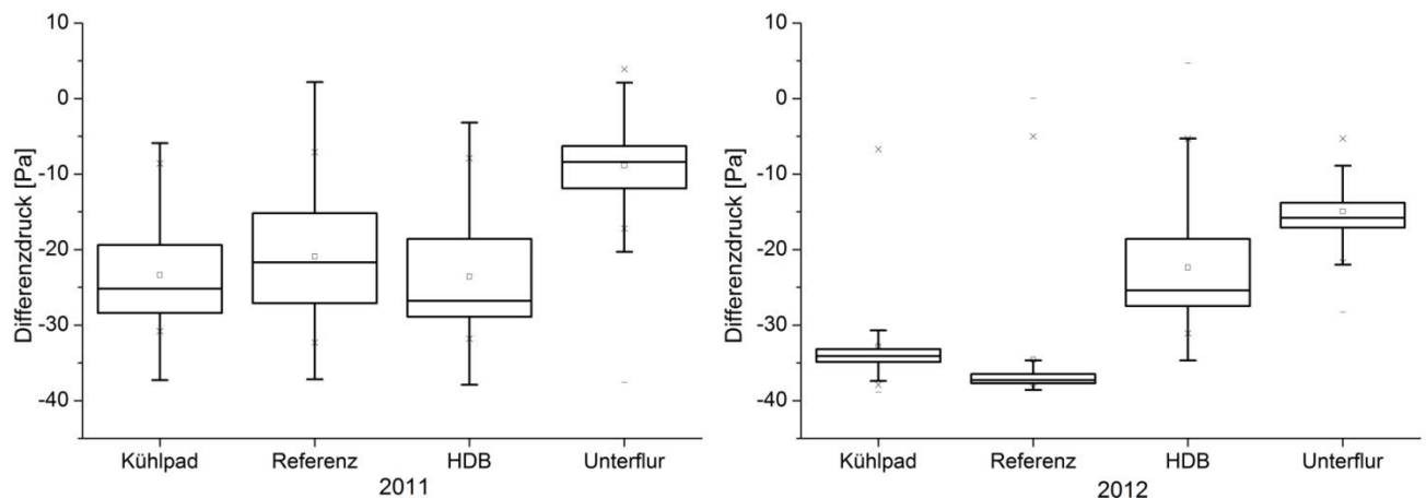
Abb. 53: Werte der Differenzdruckmessungen über die zwei wärmsten Zeiträume. Links: 18.08. – 26.08.2011 n > 25000 ; rechts: 17.08. – 21.08.2012 n > 14000
