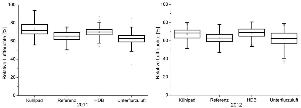
Abb. 42: Tagesdurchschnittswerte der relativen Luftfeuchtigkeit. Links: Jahr 2011 Jan. – Dez. n > 200 d, rechts: Jahr 2012 Jan. – Sep. n > 175 d. (HDB = Hochdruckbefeuchtung)
