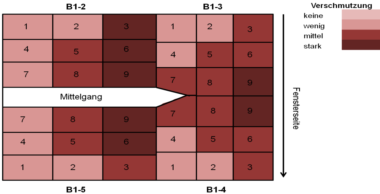
Abb. 75: Ø Buchtverschmutzung (Bereiche 1 bis 9) über alle Beobachtungen in Abteil B1 (Kühlpad). Zusammenfassung des ersten Versuchszeitraums (12 Beobachtungstage 2011).
