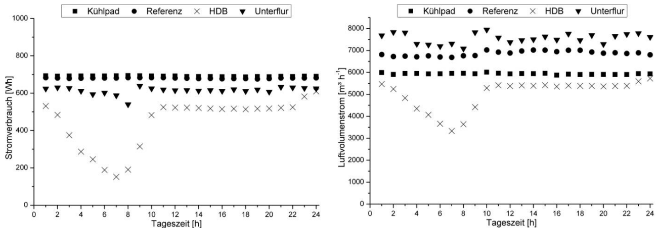
Abb. 82: Darstellung des Stromverbrauchs pro Stunde der Ventilatoren (links) und des Volumenstroms pro Stunde (rechts) vom 19. August 2012. ( \varnothing 27,4°C Außentemperatur) (HDB= Hochdruckbefeuchtung)
