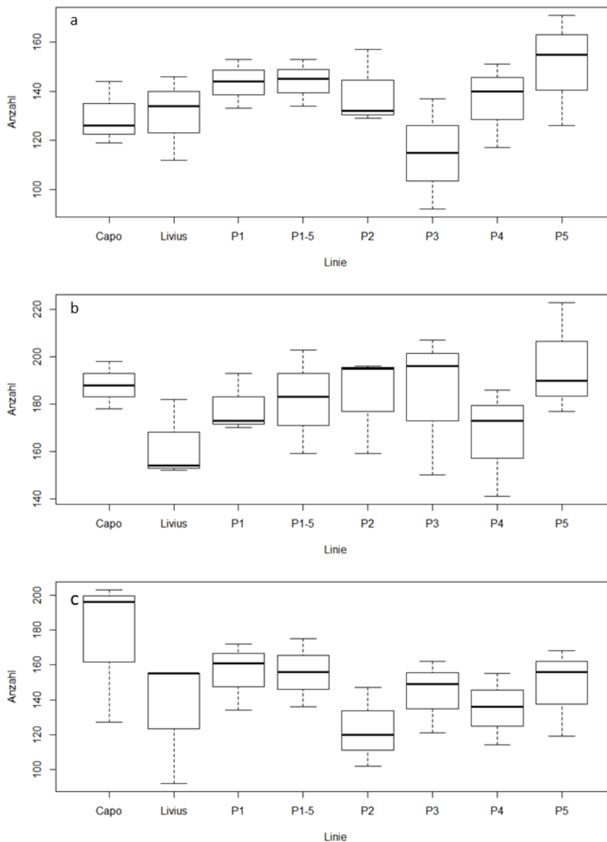
Abb. 4: Vergleich Feldaufgang aller Linien an den Versuchsstandorten Dittlofsroda (1a), Pforzen (1b) und Schwebheim (1c)
