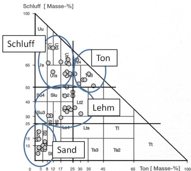
Abbildung 5.1-1: Einordnung aller untersuchten Proben in das Korngrößendreieck nach AG Bodenkunde (2005) (verändert) und deren Zuteilung zu den Bodenartenhauptgruppen.
