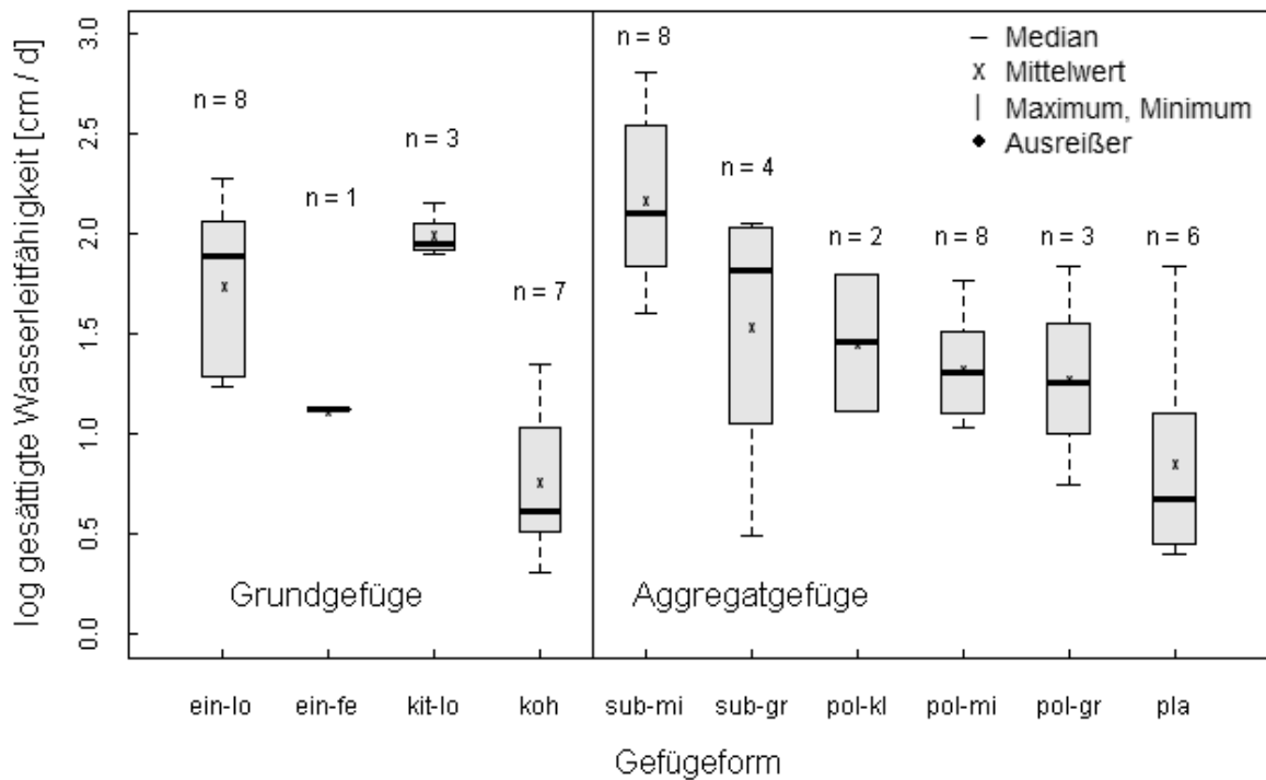
Abbildung 5.1-10: Zusammenhang der Gefügestruktur mit den logarithmierten Werten der gesättigten Wasserleitfähigkeit [ \text{cm d}^{-1} ].
