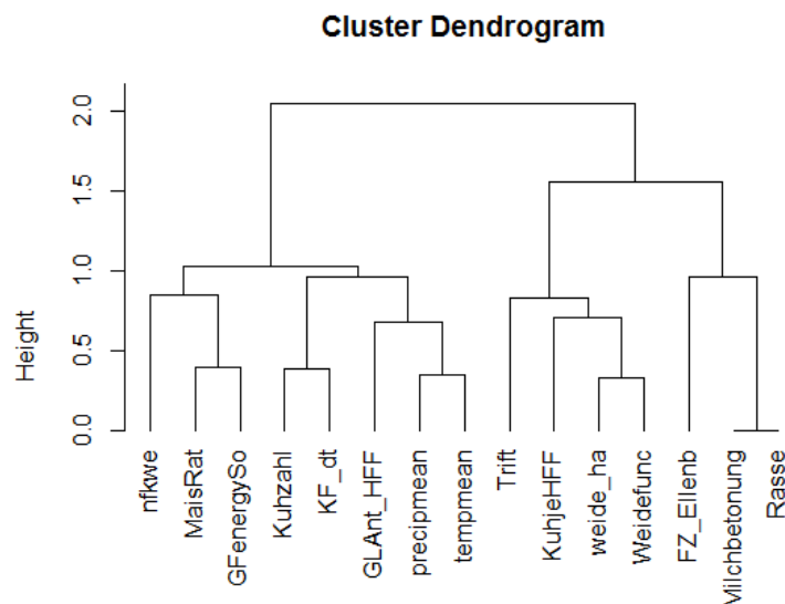
Abbildung 2: Traitcluster Dendrogram der PCAMIX (Hauptkomponentenanalyse mit unterschiedlich skalierten Variablen)
