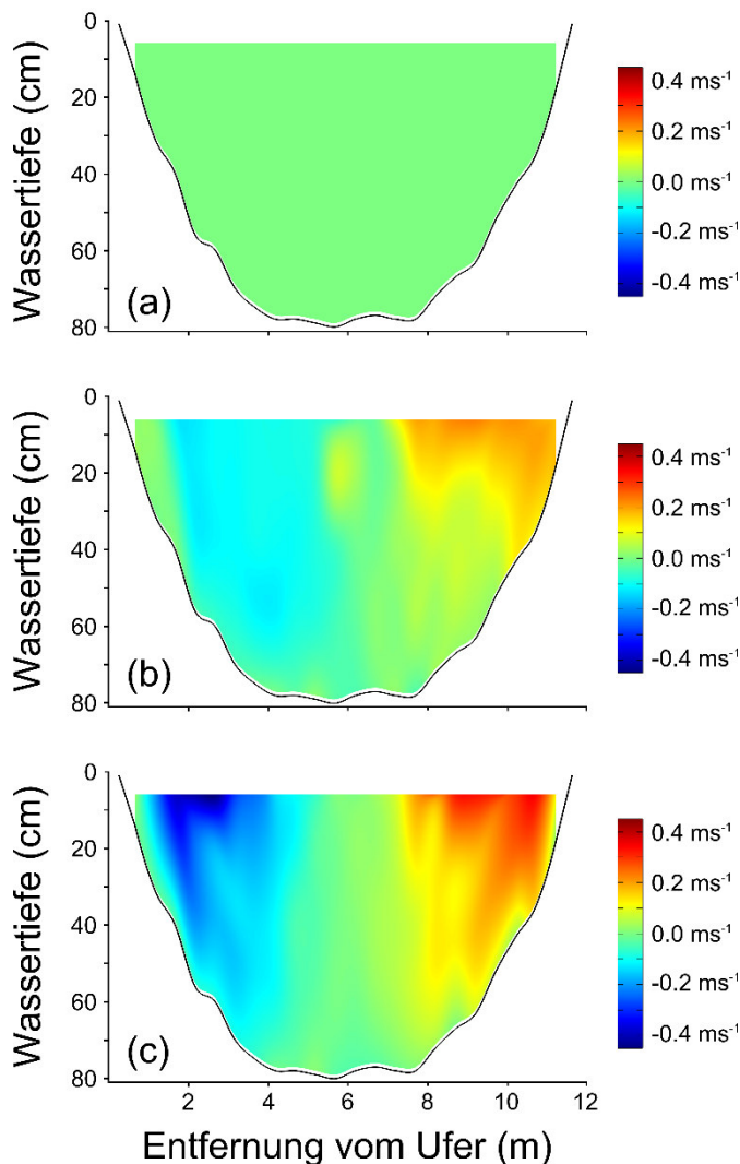
Abbildung 2: Strömungsprofile ( \text{m s}^{-1} ) in einem Erdteich (ca. 10 \times 20 m), auf dessen Wasseroberfläche zwei Schaufelradbelüfter (Motorenleistung 0,25 kW) installiert wurden. Dargestellt sind die Strömungsprofile (a) ohne Lüfter, (b) mit einem Lüfter und (c) mit zwei Lüftern im Betrieb. Negative und positive Geschwindigkeiten ergeben sich durch die erzeugte Kreisströmung. Rote Farbtöne: Strömung zum Betrachter hin; blaue Farbtöne: Strömung vom Betrachter weg.
