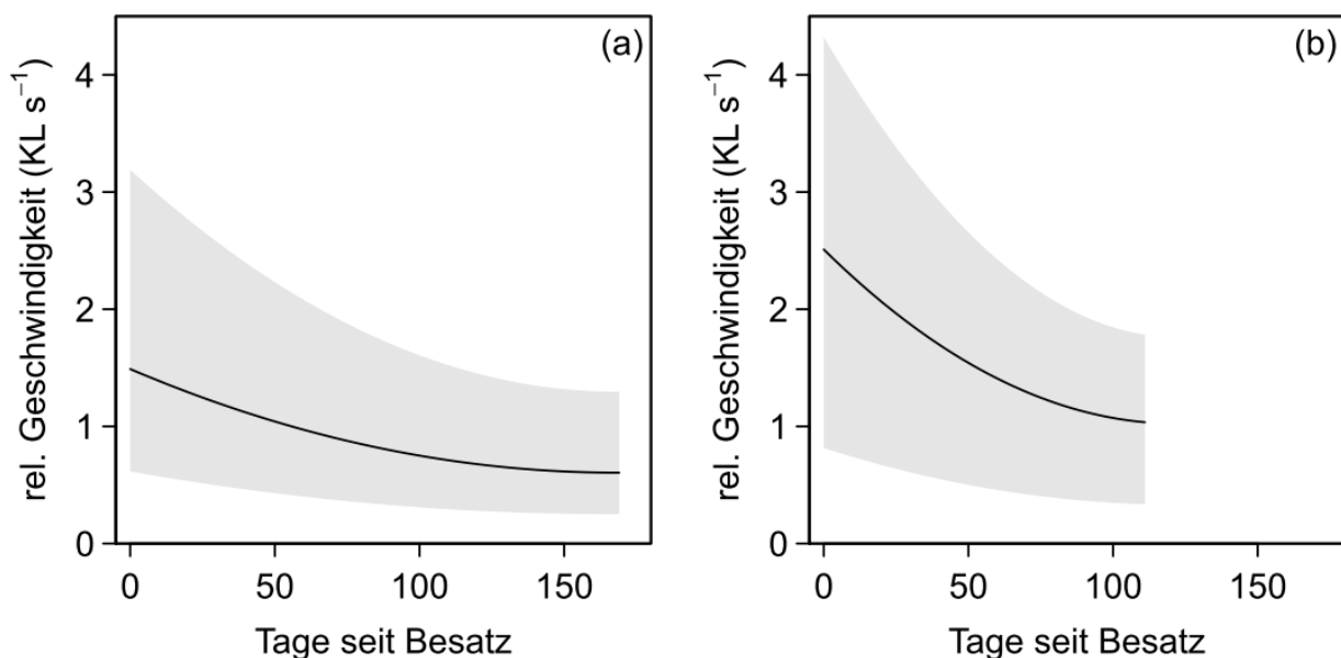
Abbildung 3: Relative Strömungsgeschwindigkeiten (angegeben als Körperlängen/Sekunde), welche durch Schaufelradbelüfter in Erdteichen erzeugt wurden. Die (a) Bachforellen wurden für 169 Tage, (b) Regenbogenforellen für 111 Tage in den Erdteichen gehalten. Die schwarze Linie stellt die mittlere Strömungsgeschwindigkeit dar, welche anhand des Median der Strömungsgeschwindigkeiten errechnet wurde. Der graue Bereich gibt die 25-75% Quantile der relativen Strömungsgeschwindigkeiten an und gibt den Bereich der zur Verfügung stehenden Geschwindigkeiten an.
